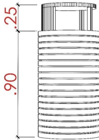
ELEVACION FRONTAL ESC: 1/100
